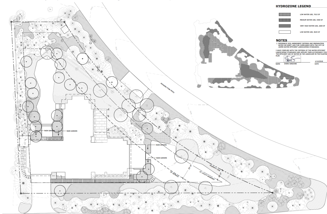
Gráfico 1B-5: Ejemplo de la zona de riego de WELS de Aspen
