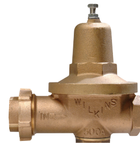
Figura 5-9: Regulador de Presión (imagen es cortesía de Zurn)
