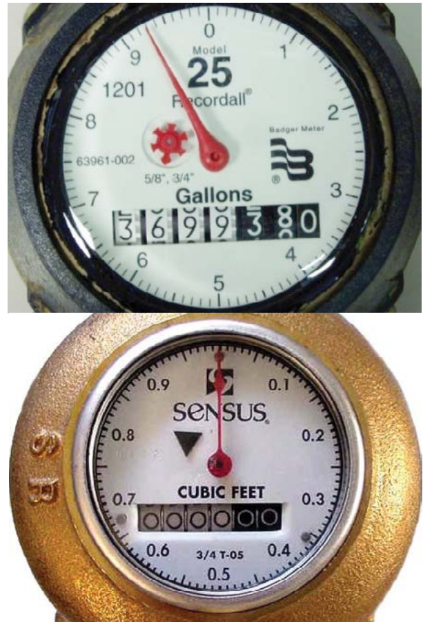
Figura 1-9: Lectura directa de medidores en galones (arriba) y pies cúbicos (abajo)
